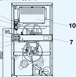
ВИД СЗАДИ Т 9 (МОДЕЛЬ С ГАЗОВЫМ НАГРЕВОМ)
