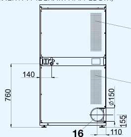
ВИД СЗАДИ Т 9 (МОДЕЛЬ С ЭЛЕКТРИЧЕСКИМ НАГРЕВОМ)
