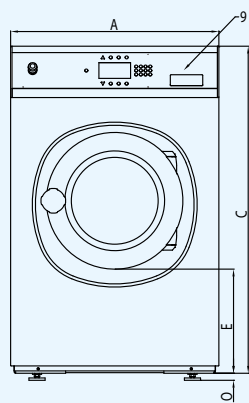
Вид спереди
